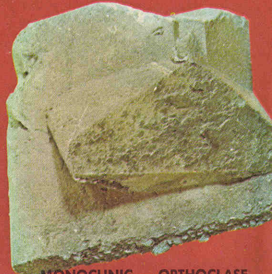
MONOCLINIC — ORTHOCLASE
